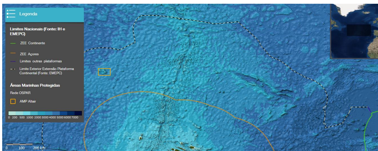
Figura 8. Área Marinha Protegida OSPAR Monte Submarino Altair. Fonte: Geoportal “Mar Português” [7]
