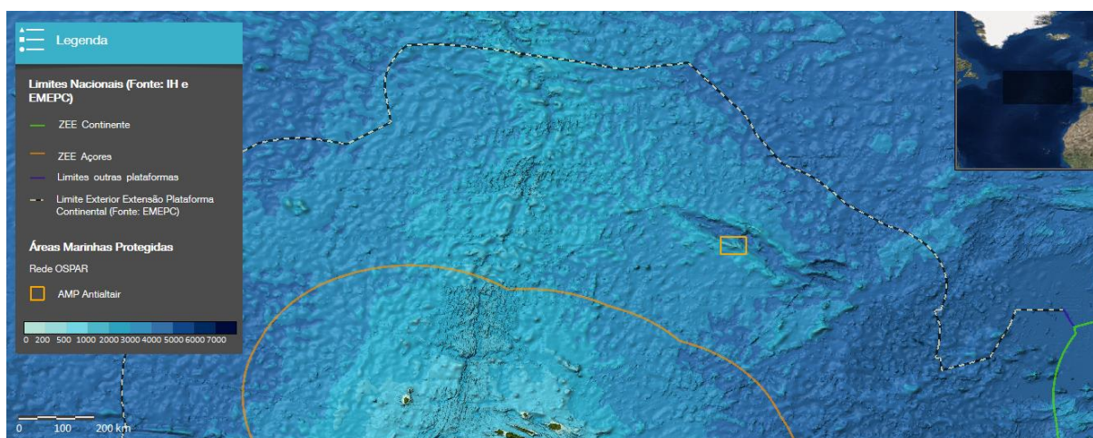
Figura 9. Área Marinha Protegida OSPAR Monte Submarino Antiltair. Fonte: Geoportal “Mar Português” [7]
