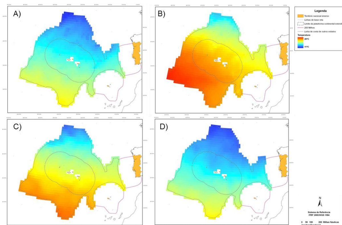
Figura 12. Média sazonal da temperatura superficial das águas sobrejacentes à subdivisão da Plataforma Continental Estendida na primavera (A), verão (B), outono (C) e inverno (D) de 2011. Adaptado de (MAMAOT, 2012b)
