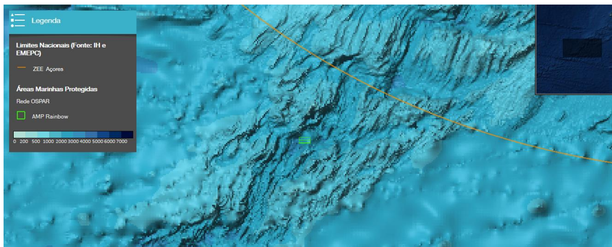
Figura 7. Área Marinha Protegida OSPAR Campo Hidrotermal Rainbow. Fonte: Geoportal “Mar Português” [7]
